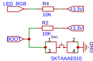
ESP32 C3
