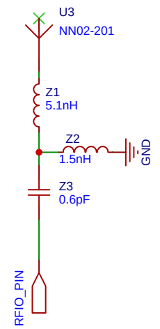
ANTENNA
