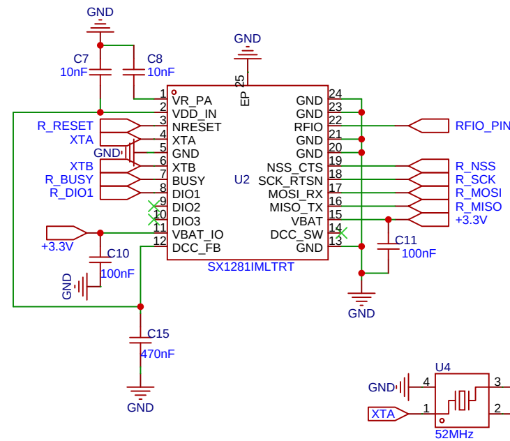
SX1281
